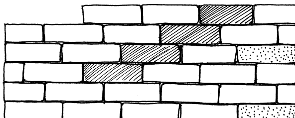
Muur in "klezoren"-verband: lopend
