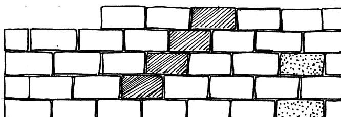
Muur in "halfsteensverband"
