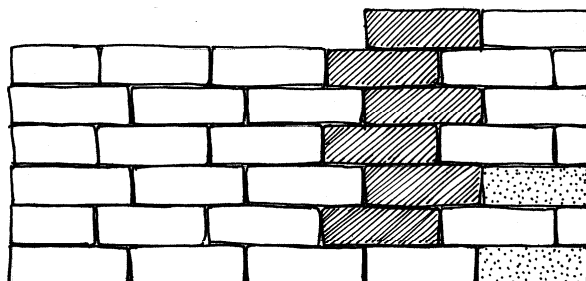
Muur in "klezoren"-verband: staand
