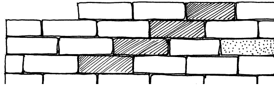
Muur in "klezoren"-verband: lopend
