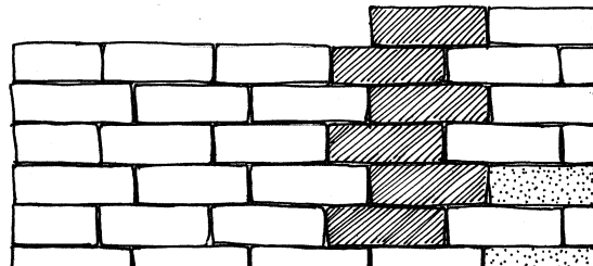
Muur in "klezoren"-verband: staand
